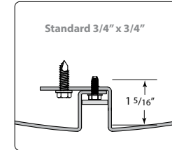
VOR Vertical Open Reveal
